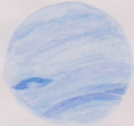
Neptun
