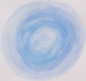
Uranus
